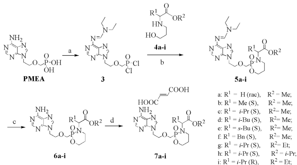
Scheme 1. Reagents and conditions: (a) (i) \text{Et}_2\text{NCHO} , (\text{COCl})_2 , \text{CH}_2\text{Cl}_2 , reflux, 3 h, (ii) \text{Py} , 0^\circ\text{C} , 20 min; (b) \text{TEA} , \text{CH}_2\text{Cl}_2 , -78^\circ\text{C} ; (c) \text{AcOH} , reflux, 2 h; (d) fumaric acid, \text{MeCN} , reflux, 1 h.
